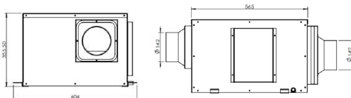
Размеры, мм
