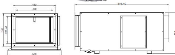
Размеры, мм
